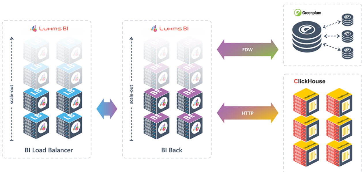
Рис. 1.7 Пример горизонтального масштабирования
